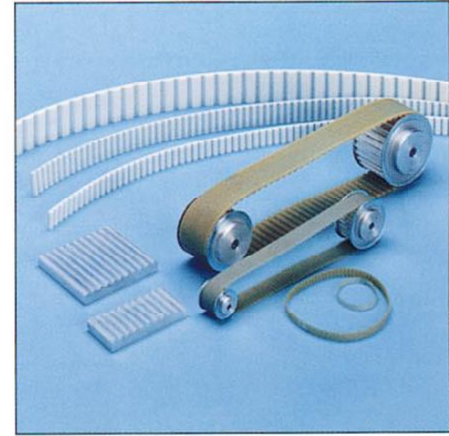
PU-hammashihnakäytöt
