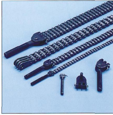
Levykimppuketjut
